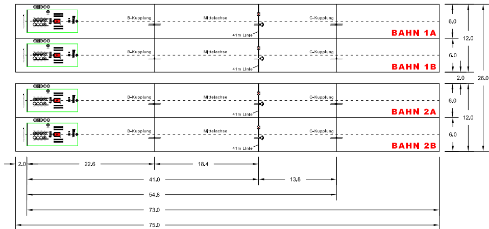
Abb. E07: Skizze für den Aufbau von zwei Bewerbsbahnen (ÖBFV)
