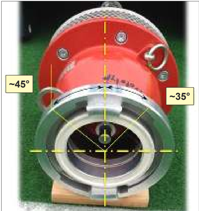
Abb. E01: Beschaffenheit Saugkorb (ÖBFV)
