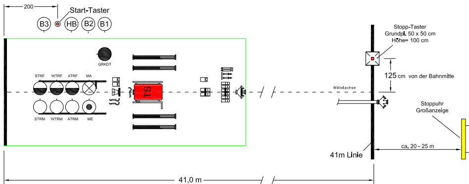
Abb. 63: Aufbau der elektronischen Zeitnehmung (MMst. Harry Simeoni)
